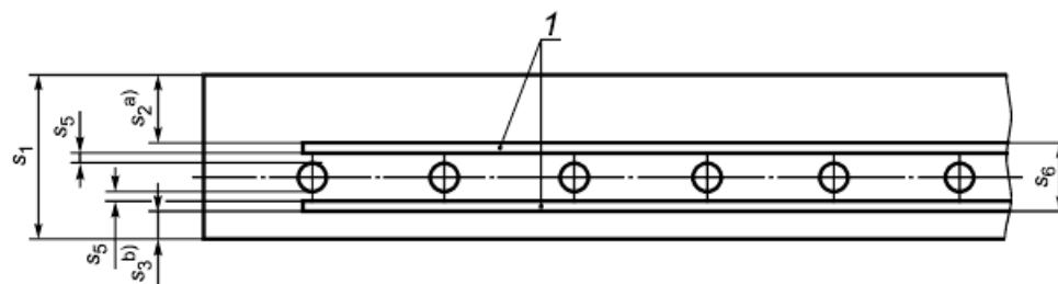
Рисунок 2 - Поперечное сечение ленты с брекером
