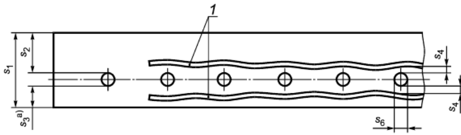
Рисунок 1 - Поперечное сечение ленты стандартного типа
